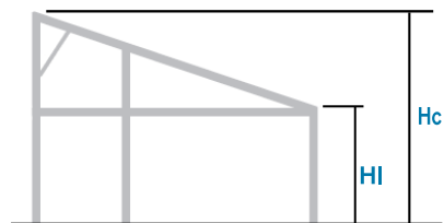
Capriata di facciata
